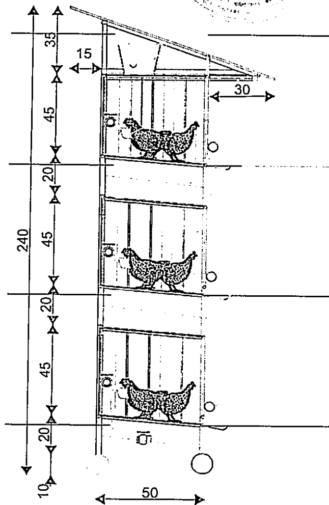
Figure 3 : B Coupe B-B.
